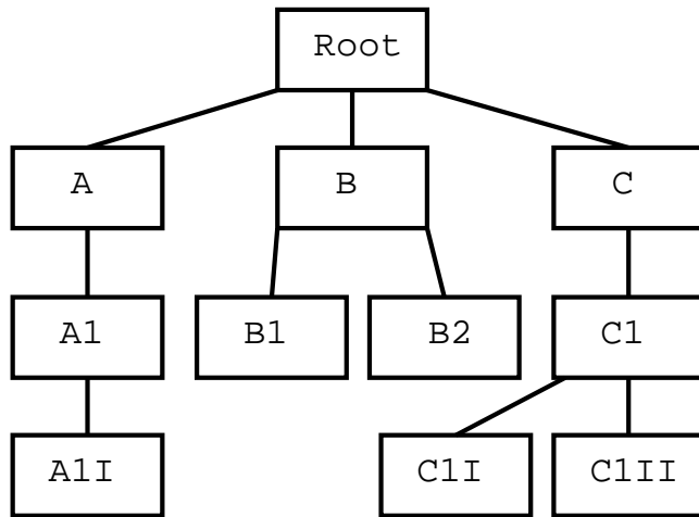
Abbildung 7.1: Unser Baum-Beispiel
