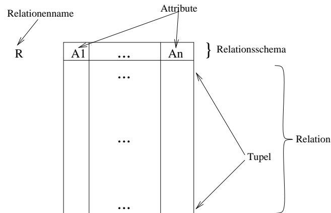
Abbildung 3.3: Tabellenstruktur
