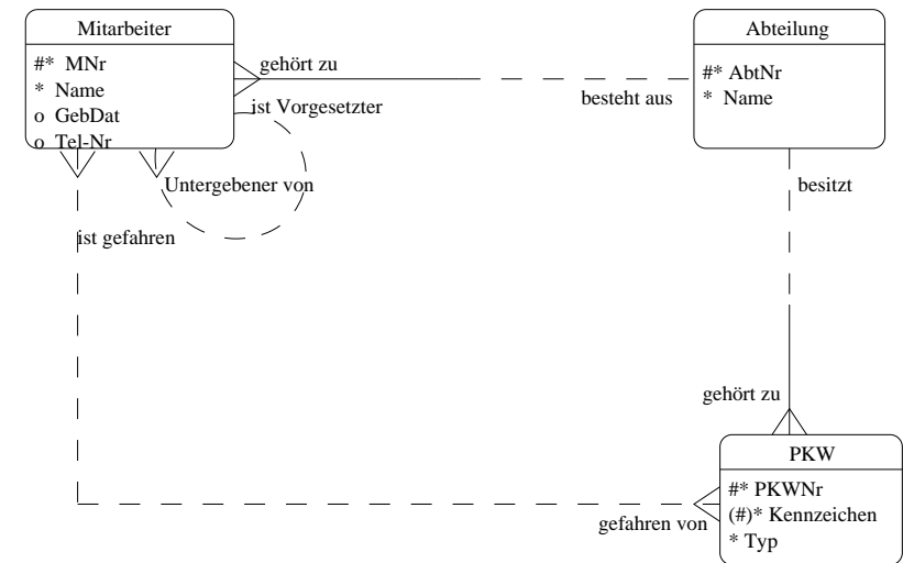
Abbildung 4.2: ER-Beispiel 1
