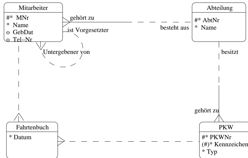
Abbildung 4.3: ER-Beispiel 2
